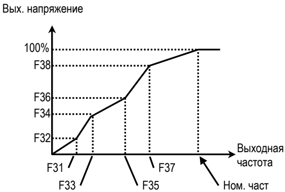
[Специальная U/F-характеристика]
