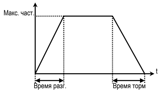
Выходная частота
