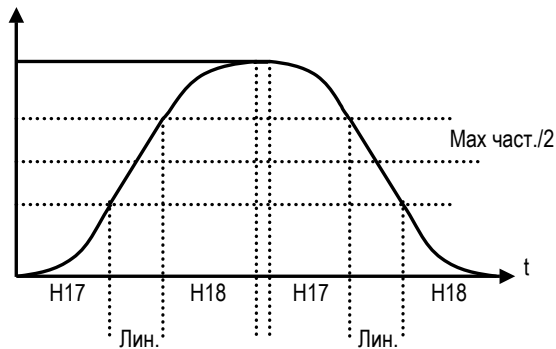
[Настройка S-характеристики]
