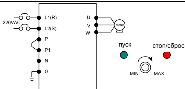
Схема подключения
